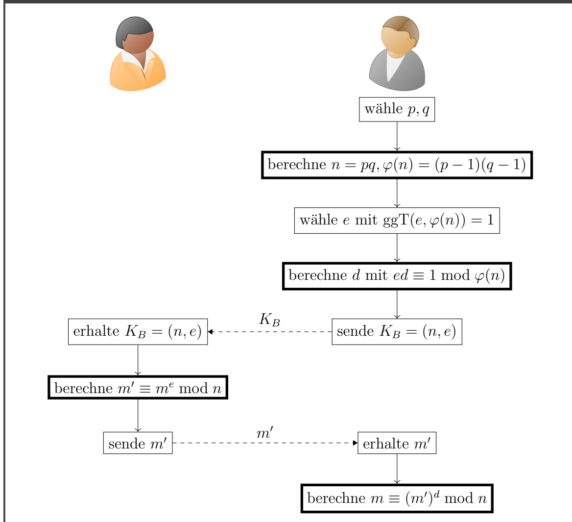
Abbildung 12: RSA-Verschlüsselung
